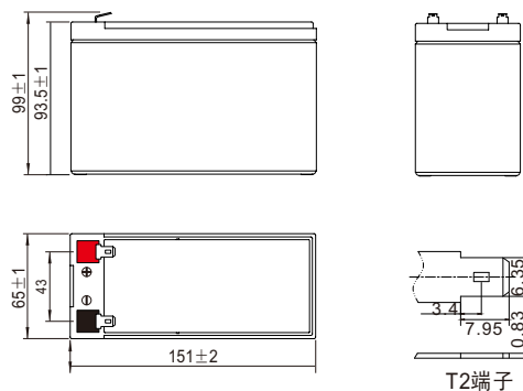
T2端子
