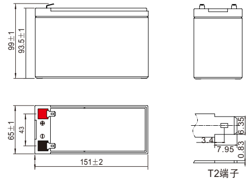
T2端子
