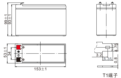
T1端子
