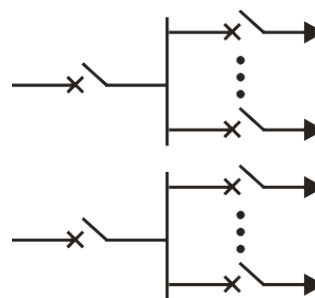
双母线系统
