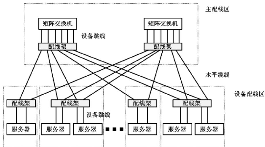
图11 前端网络布线系统基本结构图（二）
