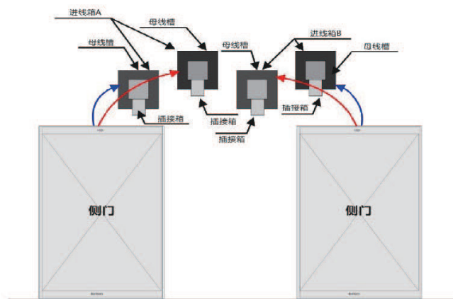
侧面示意图
